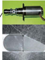
Oリング&テーパバック (高圧用シール構造)
